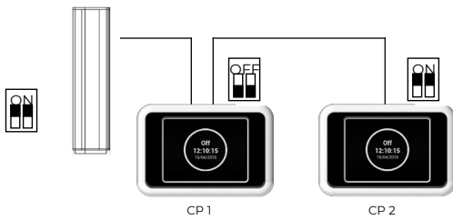
Elektrické zapojení - Možnost 1:
