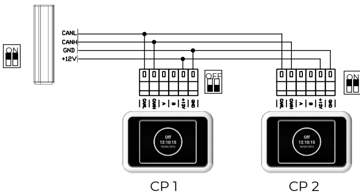
Elektrické zapojení - Možnost 1:
