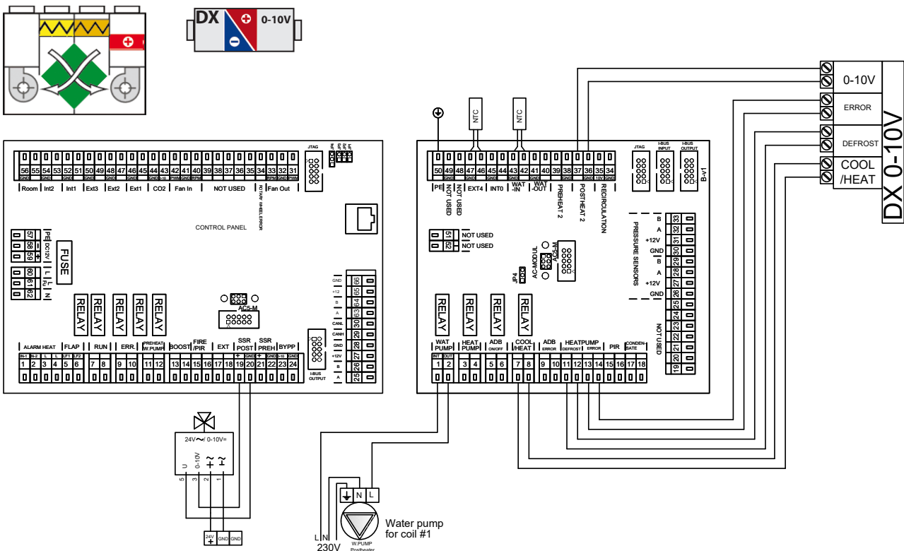
jednotka s vodním výměníkem a druhým externím výměníkem DX s regulací 0-10V
